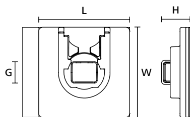
SMB4APT-A
