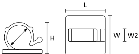
RA3-RA18- kaapelikiinnikkeet
