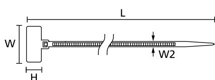
IT18FL
