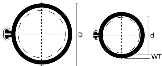
RMS-korjauskääre, liimallinen
