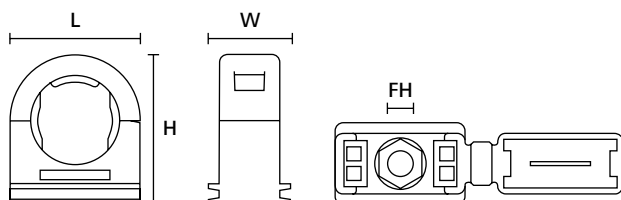
Suojaletkukiinnike sivusta
