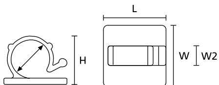
RA3-RA18- kaapelikiinnikkeet
