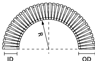
Terässuojaletku suojavaipalla
