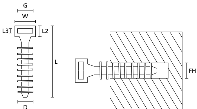
LOK01-ja LOK01B-johdinsideankkurit
