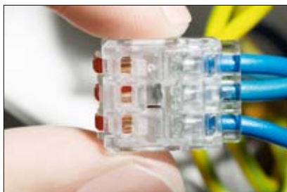
Liittimen läpinäkyvä runko mahdollistaa asennuksen tarkistuksen.
